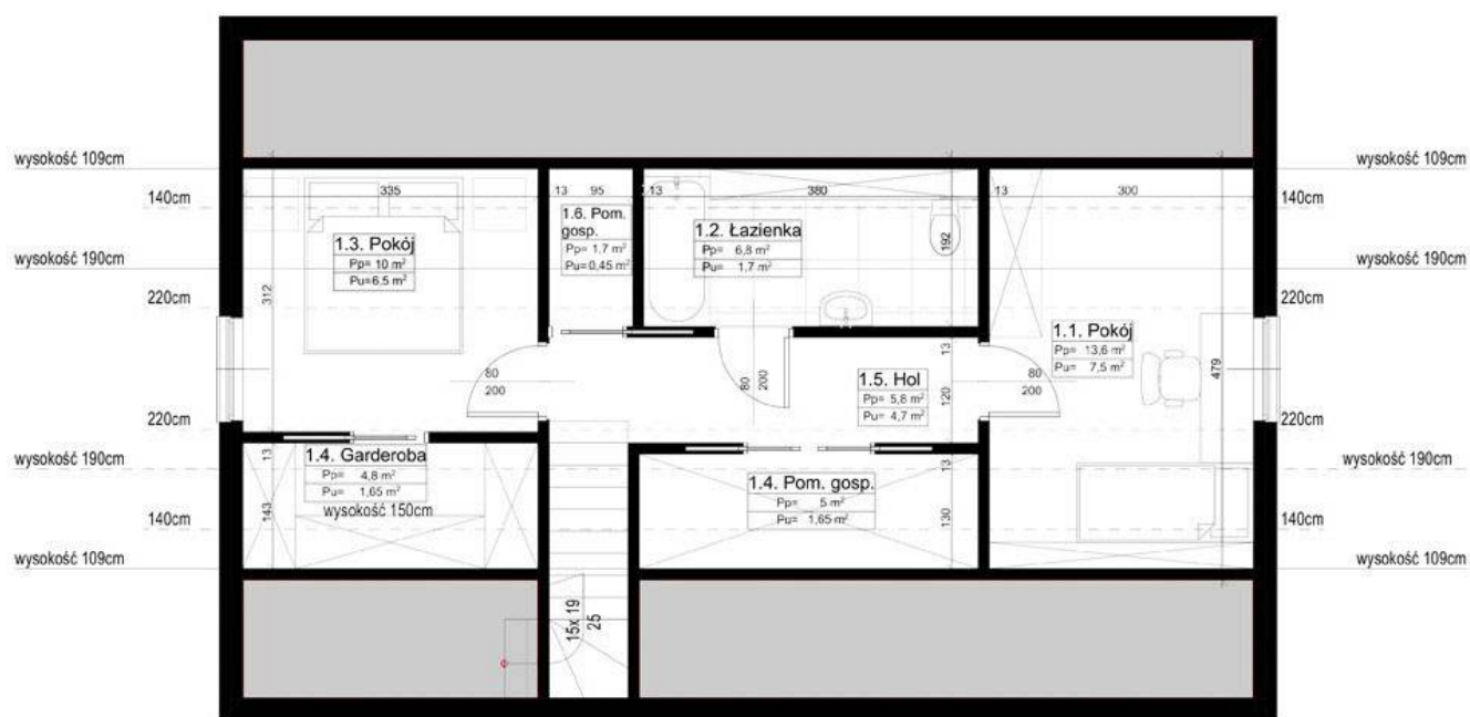
Projekt ERDOL 3 - Wersja prawa (salon po prawej stronie) - Adaptacja poddasza - przykładowa propozycja układu funkcjonalnego
