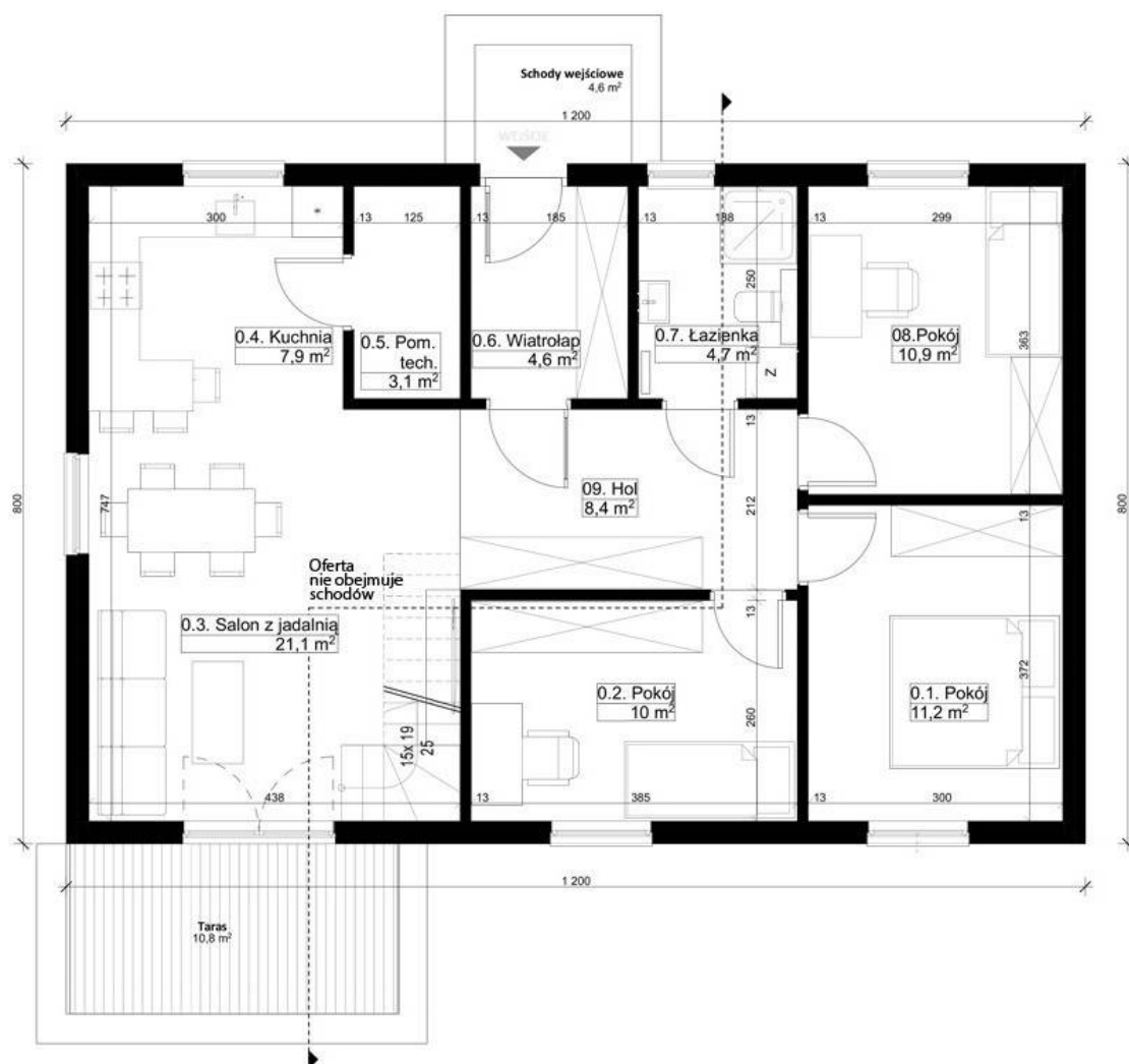
Projekt ERDOL 3 - Wersja prawa (salon po prawej stronie) - Rzut parteru
