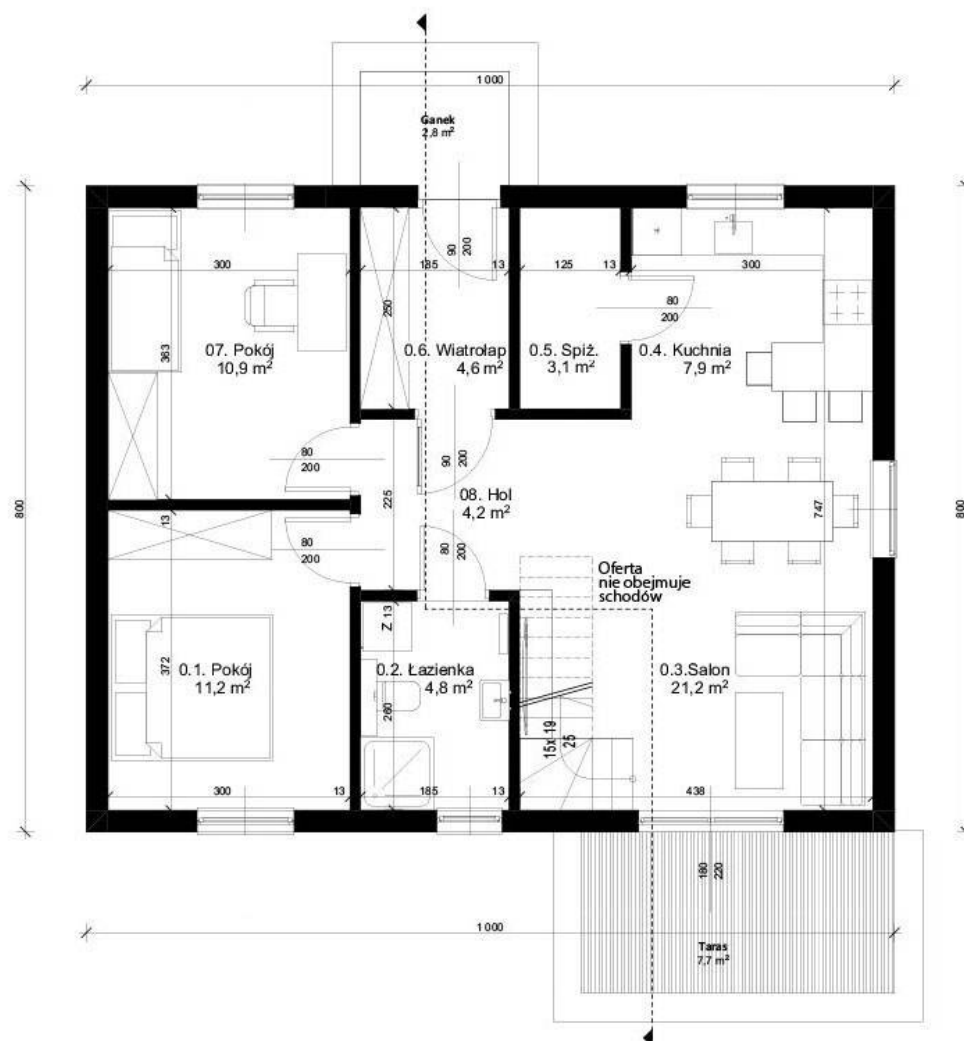
Projekt ERDOL 2 - Wersja lewa (salon po lewej stronie) - Rzut parteru
