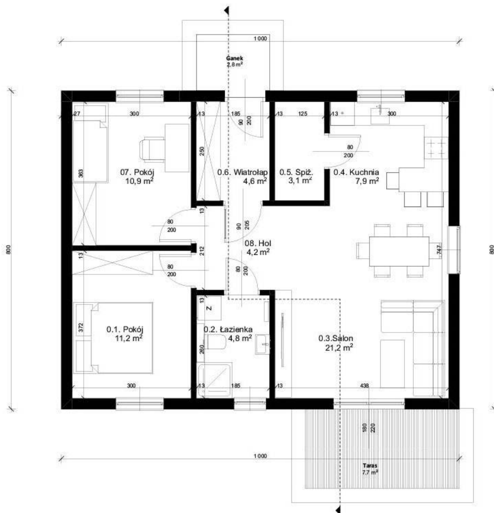
Projekt ERDOL 2 - Wersja lewa (salon po lewej stronie) - Rzut parteru
