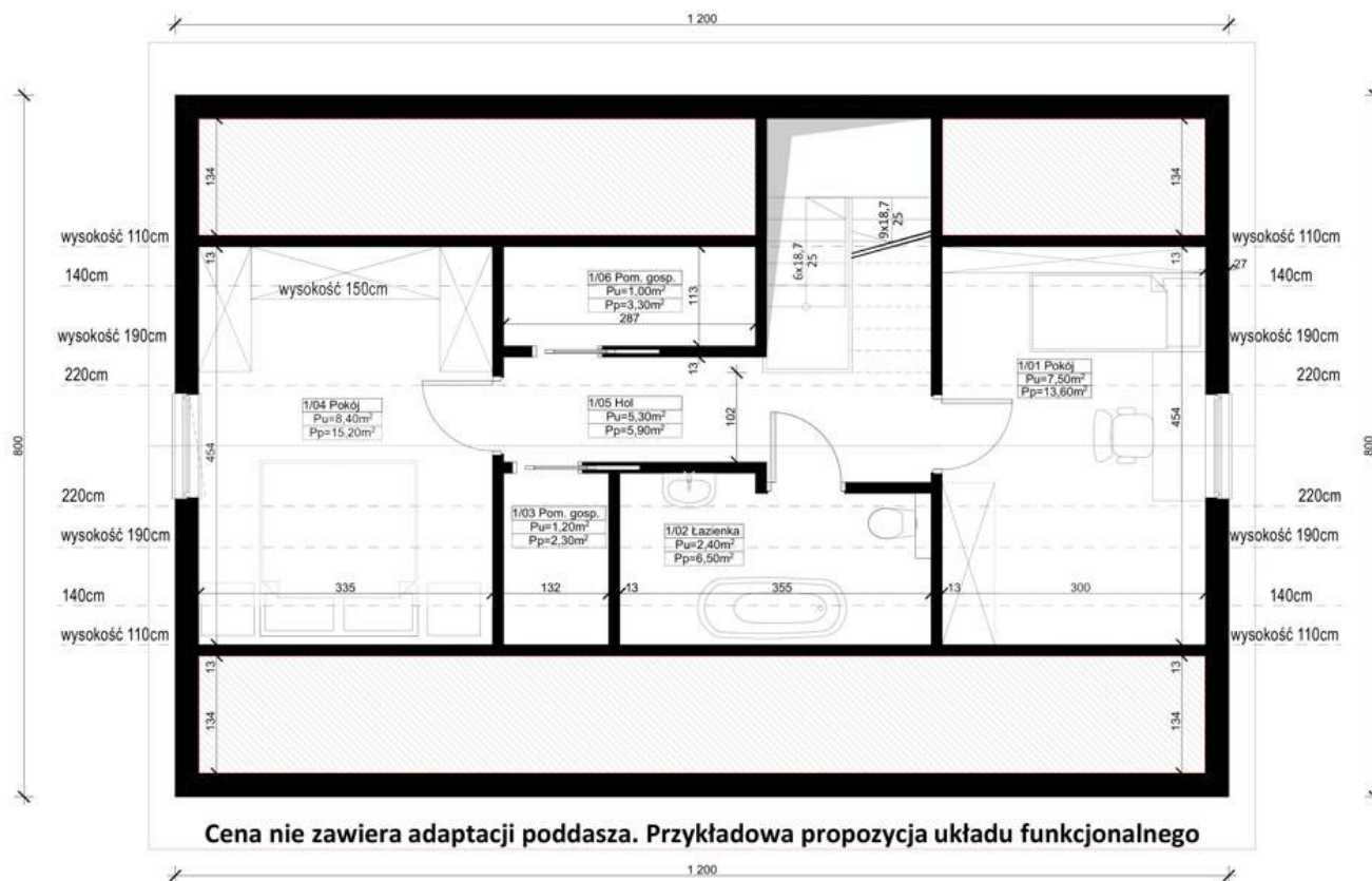
Projekt ERDOL 2 XL - Wersja prawa (salon po prawej stronie) - Adaptacja poddasza - przykładowa propozycja układu funkcjonalnego
