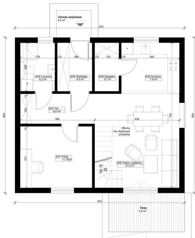
Projekt ERDOL 1 - Wersja lewa (salon po lewej stronie) - Rzut parteru
